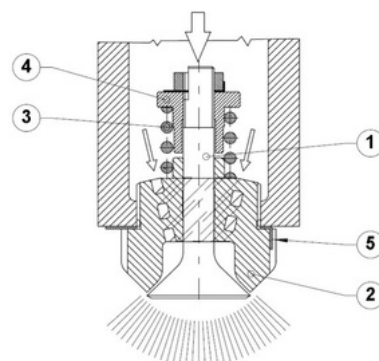
噴水減溫噴頭系列
