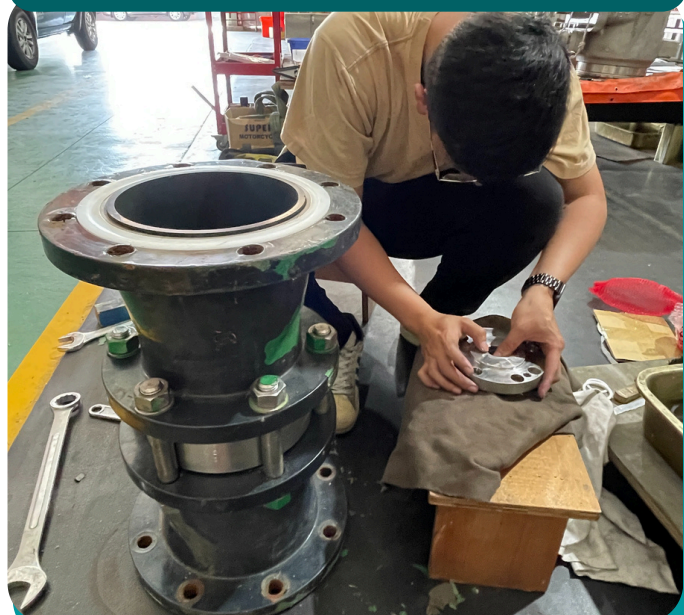
陶瓷閥整修
