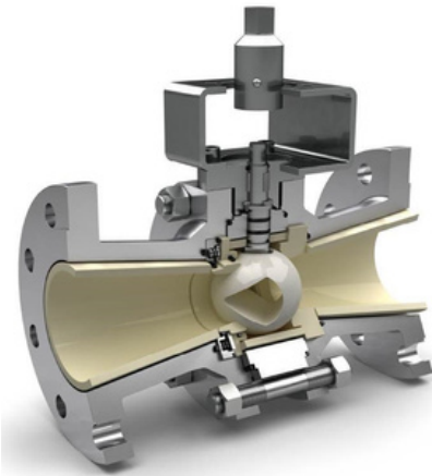
KST type: 全不鏽鋼襯陶瓷
