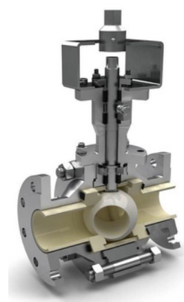
KST-HT: 高溫型陶瓷閥
